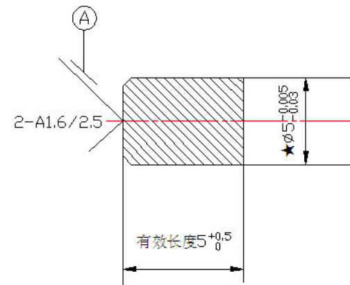
配套电机轴
