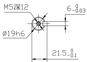
输出轴
